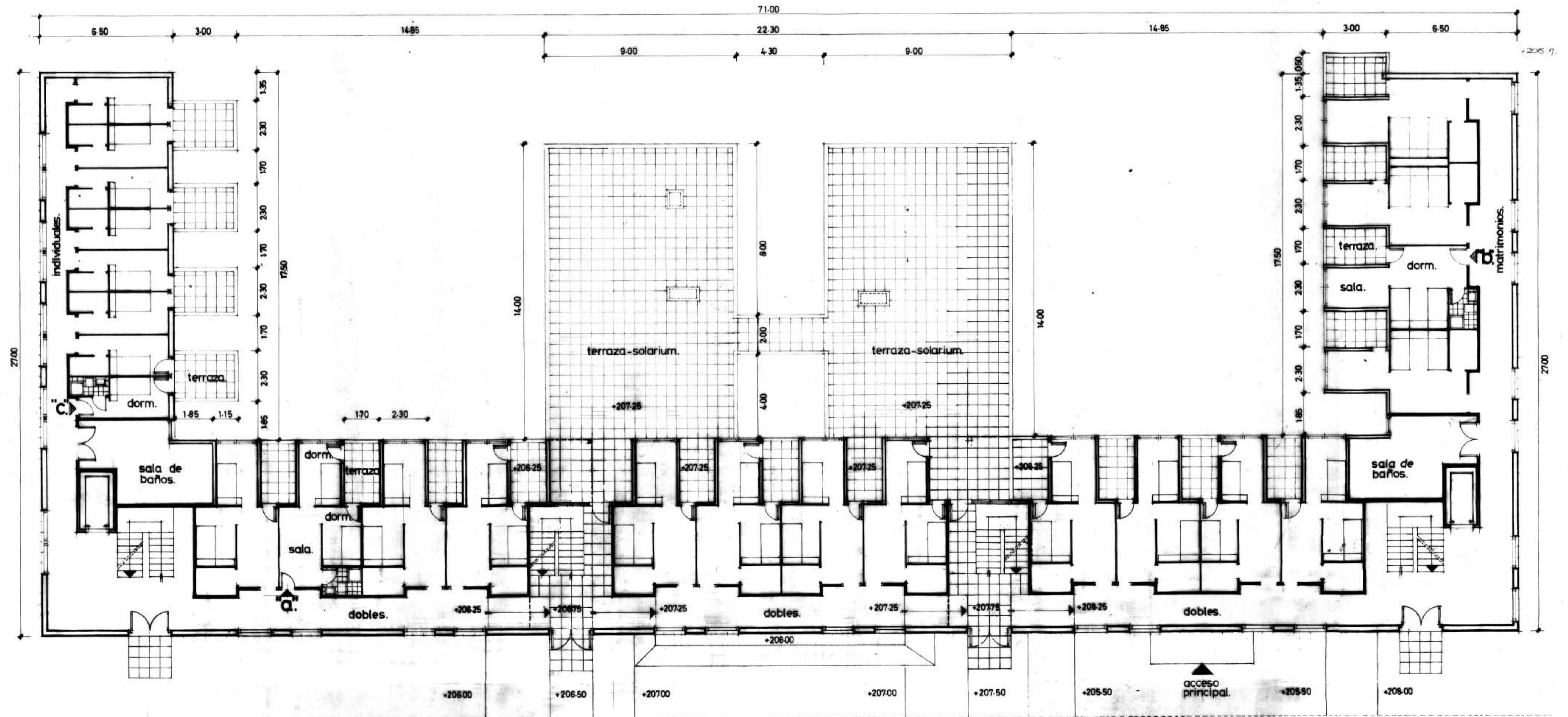
planta primera. sup. construida: 857.00 m 2 .
